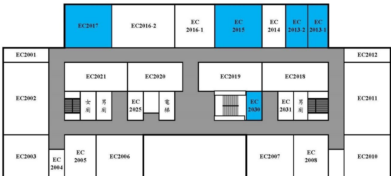
國立中山大學電資大樓二樓平面圖
